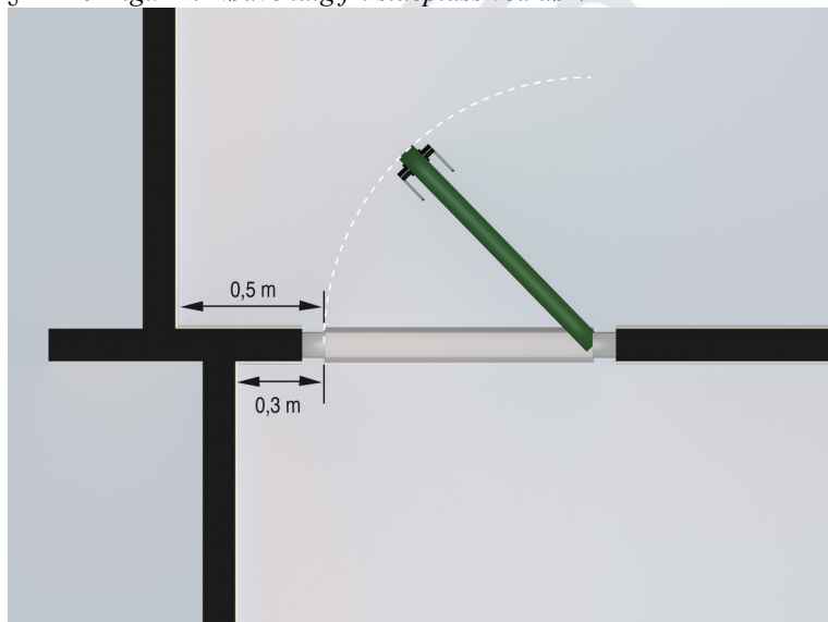
§ 12-15 Figur 2: Nødvendig fri sideplass ved dør.
