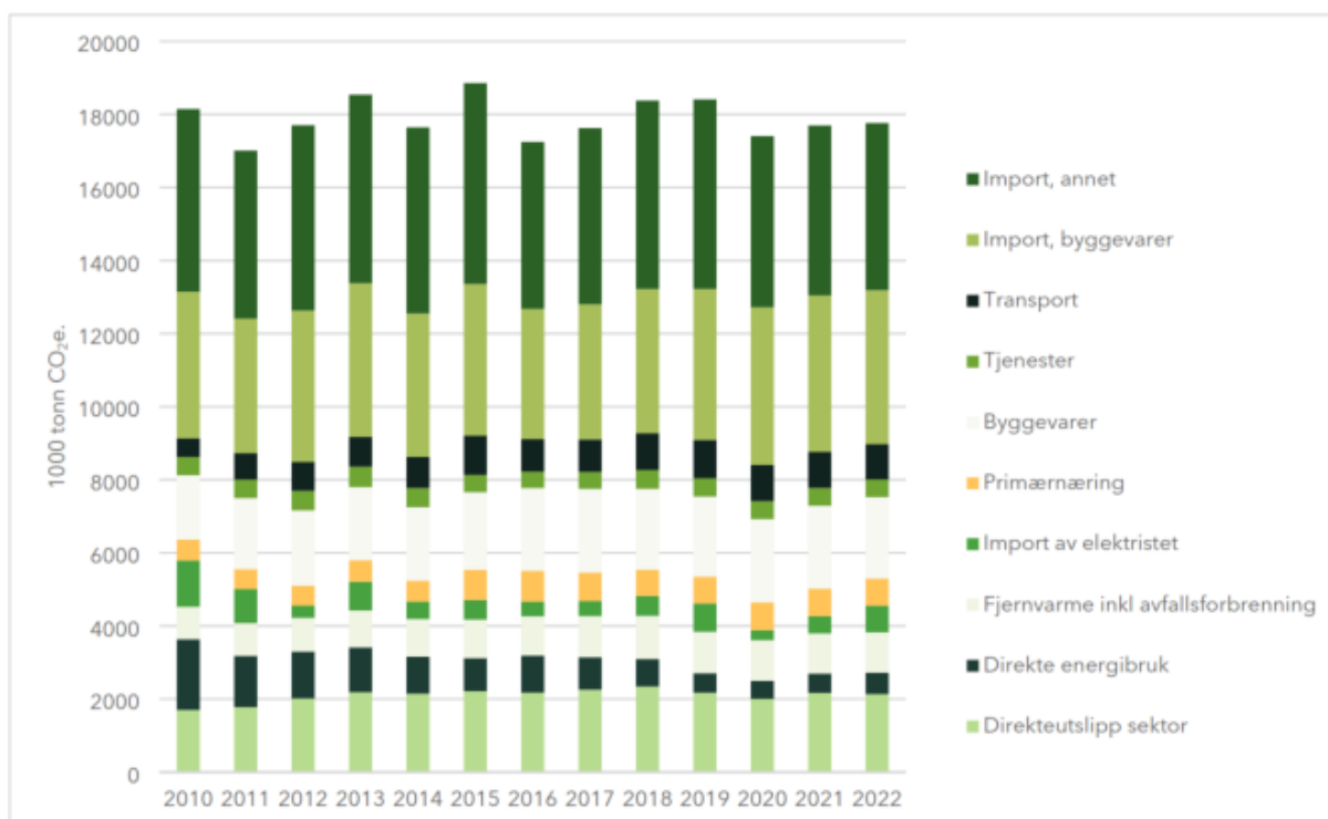
Figur 6: Klimafotavtrykk av norsk bygg- og anleggssektor
