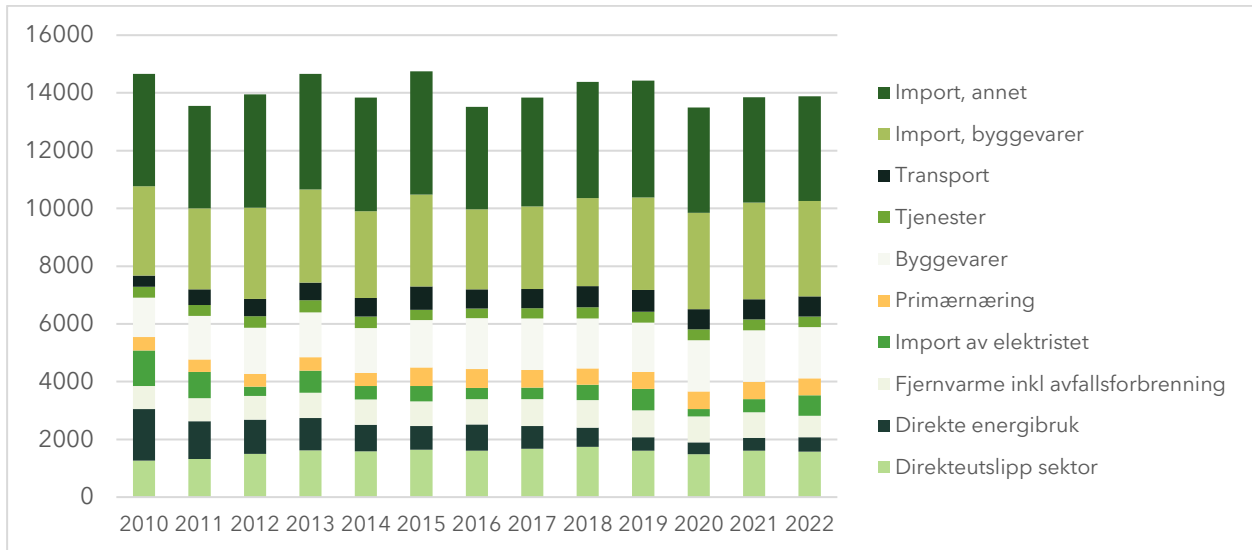
Figur 9: Klimabidrag bygg, samlet
