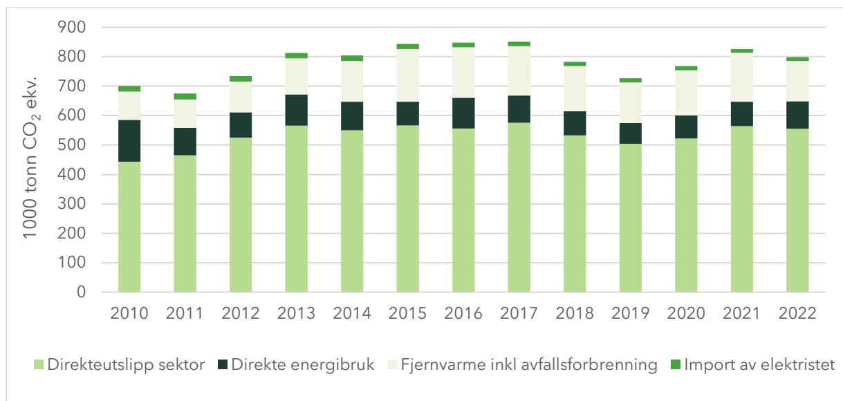
Figur 12: Klimabidrag fra direkteutslipp og energibruk, anlegg
